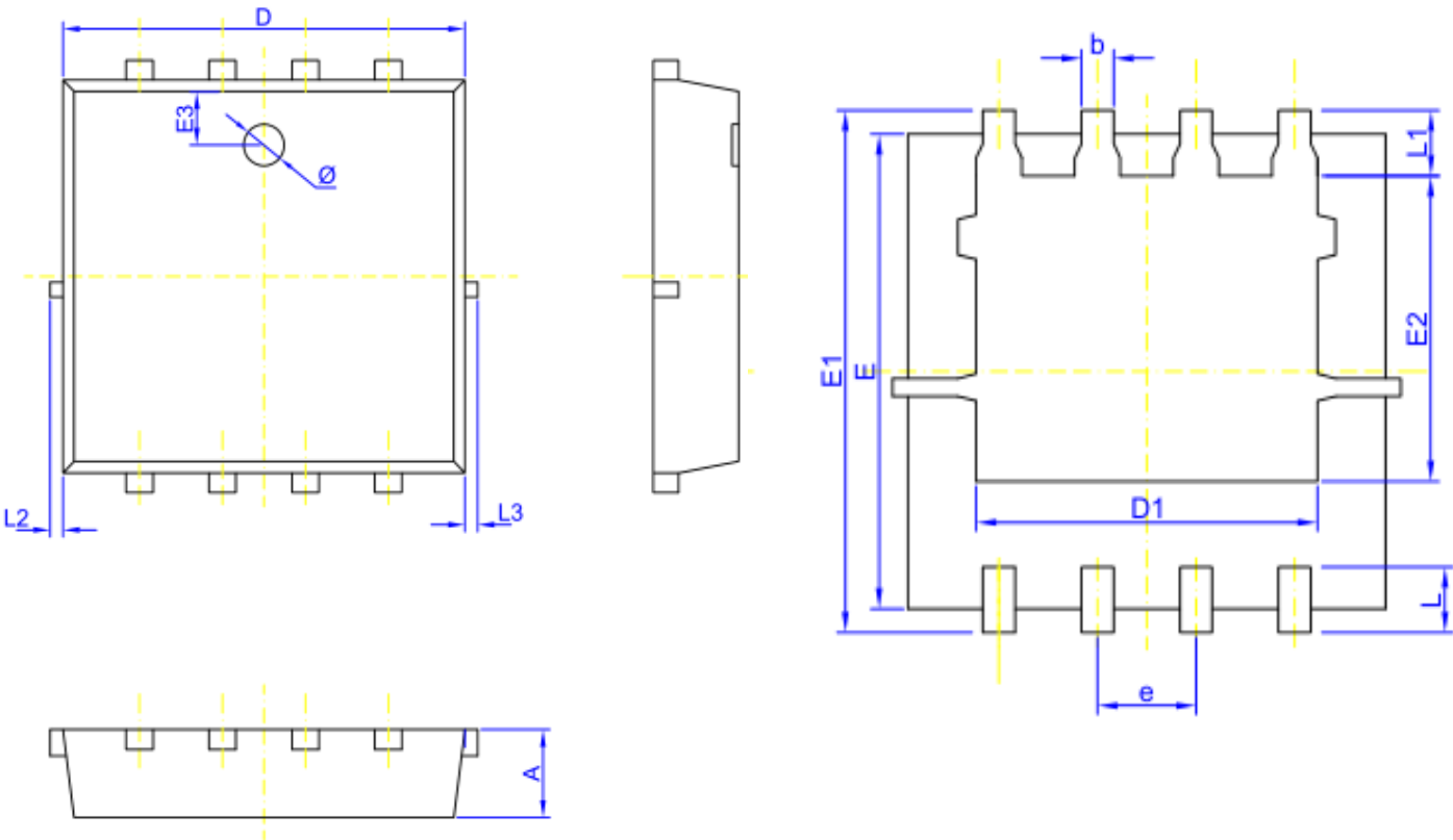
PDFN5*6 Package
